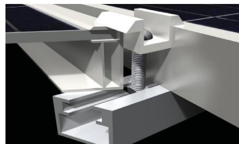
Exemple B: étrier
