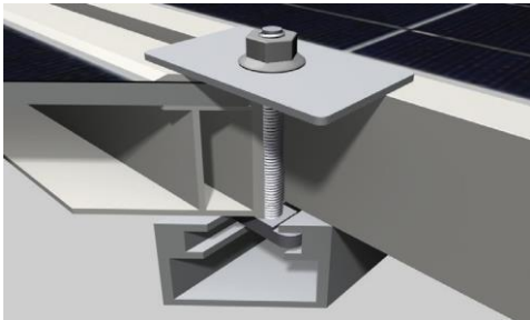
Esempio A: Morsetto a piastra
